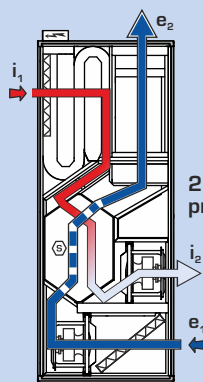
1. ventilatie cu presiune constantă si recuperarea căldurii
