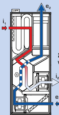
1. vienodo slėgio vėdinimas su rekuperacija
