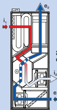
1. lige trykventilation med varmegenvinding
