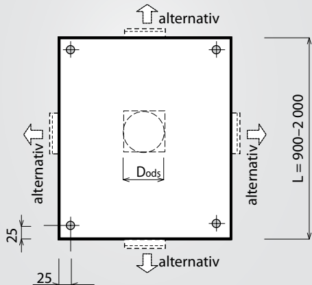
POGLED ODOZGO
