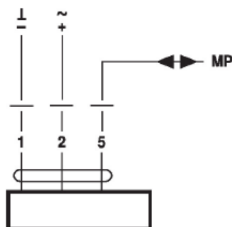
Schémata zapojení
