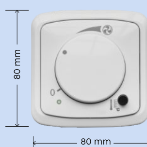
Vezérlő CPB
