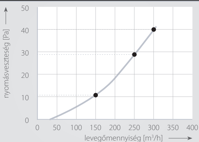
A 500×175 MM-ES LAMELLÁS SZEPARÁTOR NYOMÁSVESZTESÉGE
