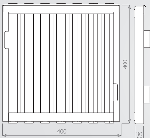
A 400×400 mm-es zsírfogó méreti ábrája
