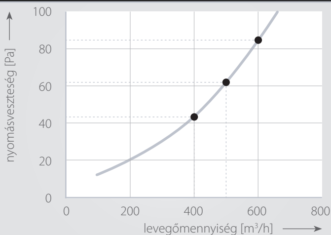
A 400×400 MM-ES LAMELLÁS SZEPARÁTOR NYOMÁSVESZTESÉGE
