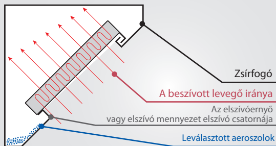
A LAMELLÁS SZEPARÁTOR FUNKCIÓJÁNAK ÁBRÁJA
