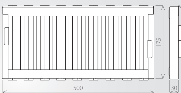
A 500×175 mm-es zsírfogó méreti ábrája
