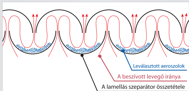
A LAMELLÁS SZEPARÁTOR FUNKCIÓJÁNAK ÁBRÁJA
