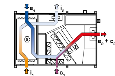
Cirkulációs fűtési és szellőztetési mód
