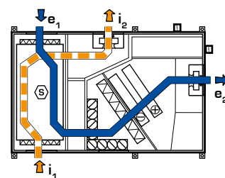
Szellőzés üzemmód hőviszanyerés nélkül (by-pass segítségével)
