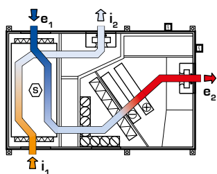
Egyenlő nyomású szellőzés
