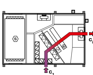
Cirkulációs fűtés üzemmód sokkos szellőzéssel
