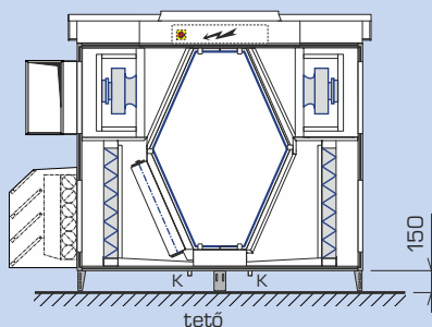
Parapet kültéri kialakítású 650-6000 Flexi
