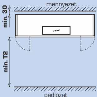
Mennyezet alatti belső 650-3500 Flexi
