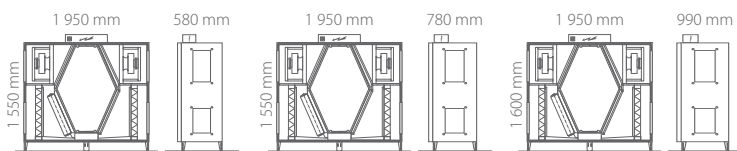
DUPLEX 2300 Flexi 3
