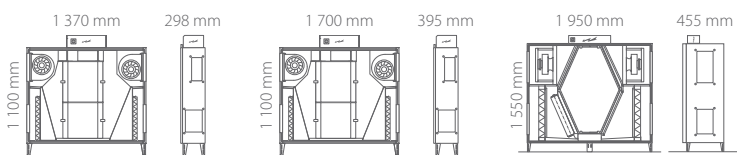
DUPLEX 650 Flexi 3
