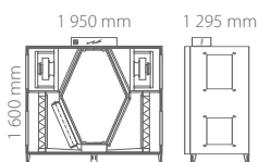
DUPLEX 6000 Flexi 3
