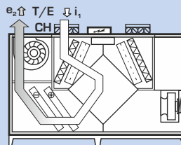
Circulatieverwarming of koeling
