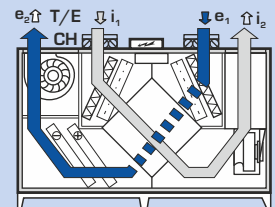
Ventilatie zonder warmteterugwinning (via bypass)
