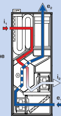
2. нощно предварително охлаждане чрез байпас през лятното часово време
