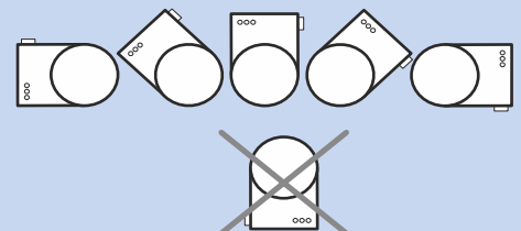
Tillatte klemmeposisjoner
