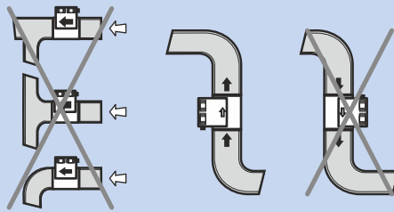
Schemat umieszczenia nagrzewnic na kanale
