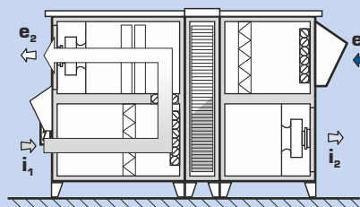
Šildymo arba vėsinimo cirkuliacija
