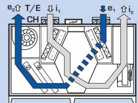
Belüftung ohne Wärmerückgewinnung (durch Bypass)
