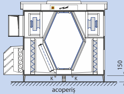
Poziție verticală pe acoperiș 650–6000 Flexi
