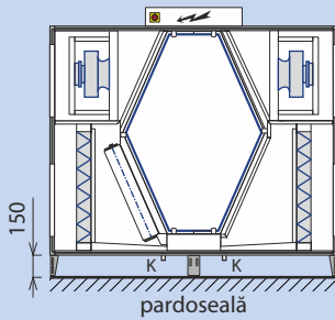
Poziție verticală pe pardoseală 650–6000 Flexi
